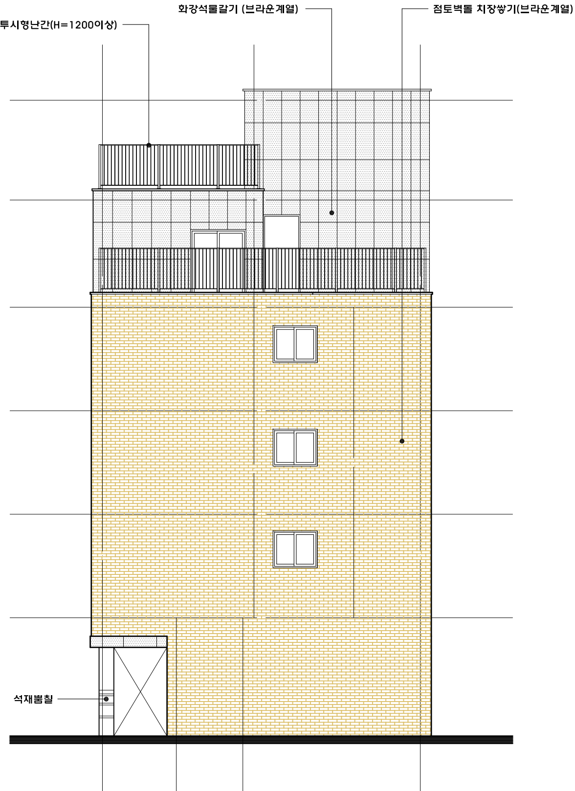
북 측 면 도 SCALE = 1/100
