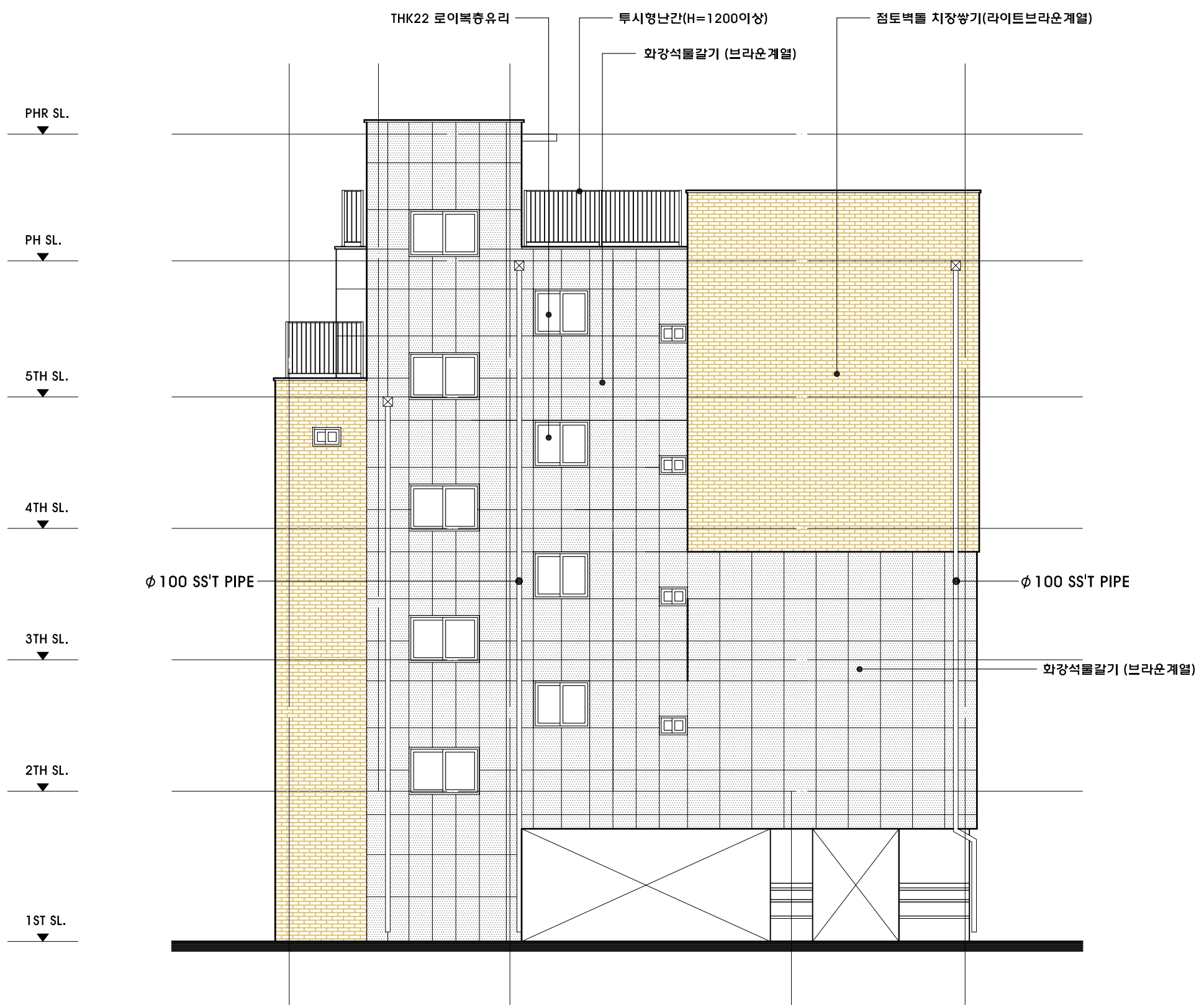
서 측 면 도 SCALE = 1/100
