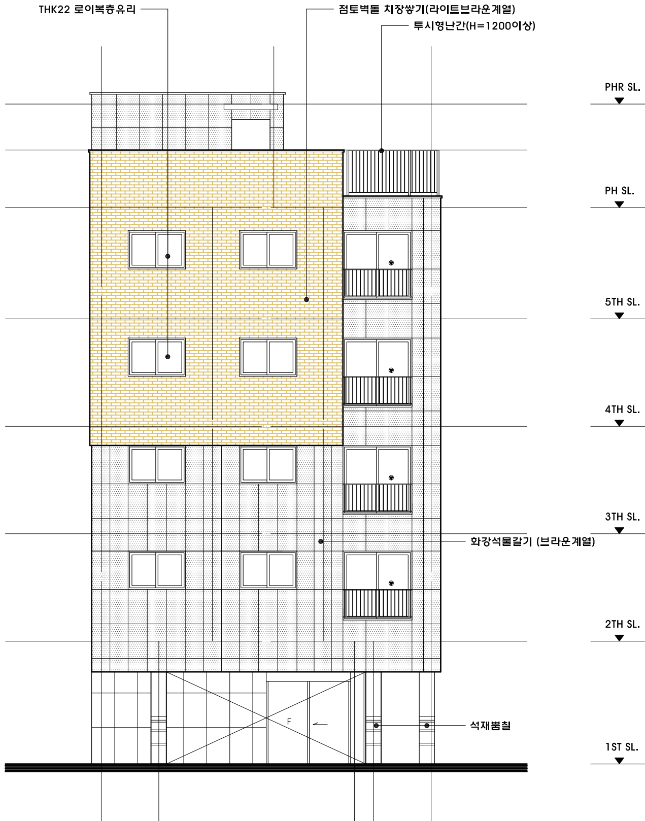
남 측 면 도 SCALE = 1/100
